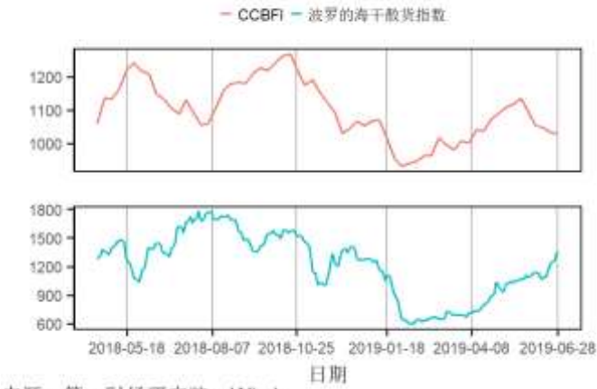
图17 中国沿海散货运价指数（CCBFI）环比下跌4.63至1028.16点，波罗的海干散货价格指数环比上涨115至1354点
